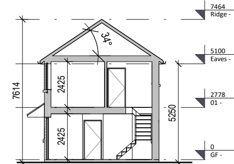
⑧ Section B-B 1 : 200
